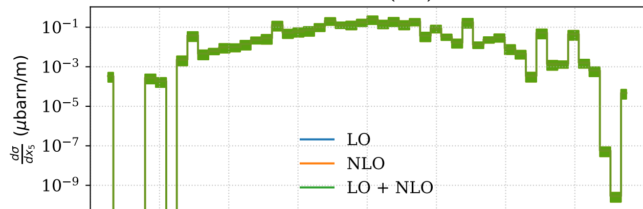
Photon x(lab)
