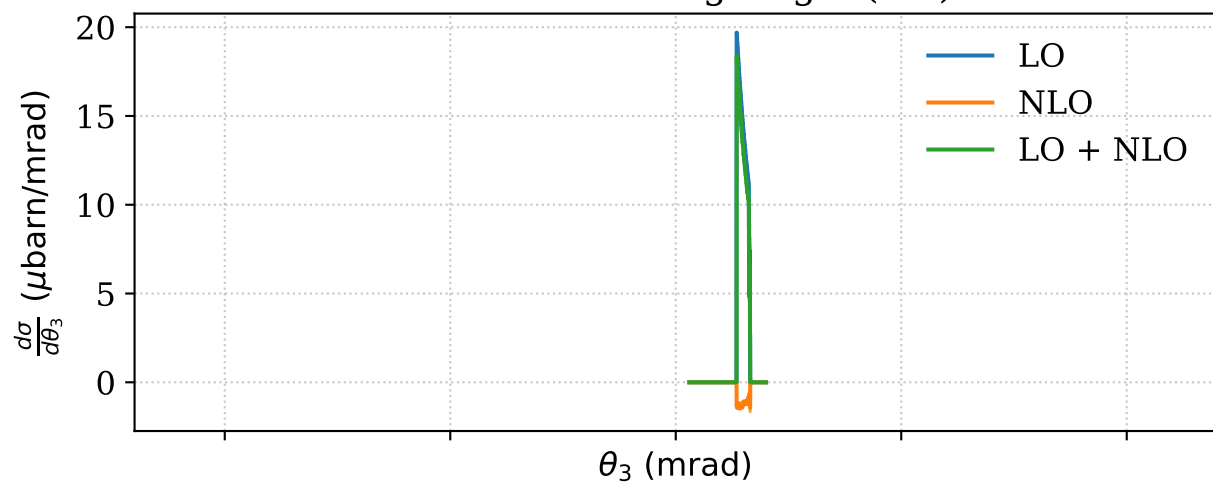
Muon Scattering Angle (lab)
