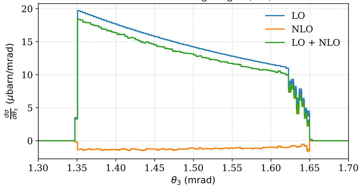
Muon Scattering Angle (lab)
