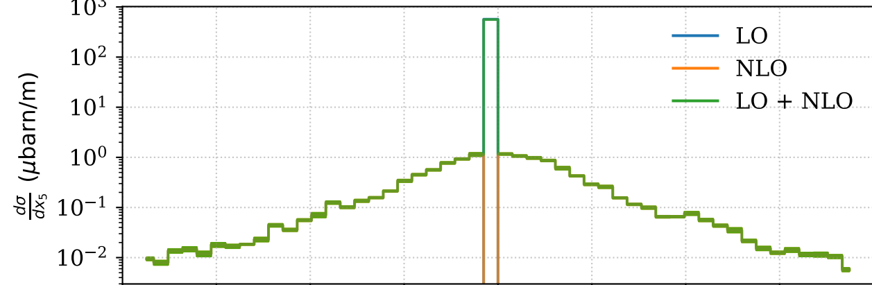
Photon x(lab)
