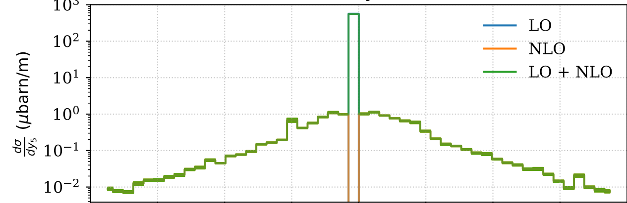
Photon y(lab)
