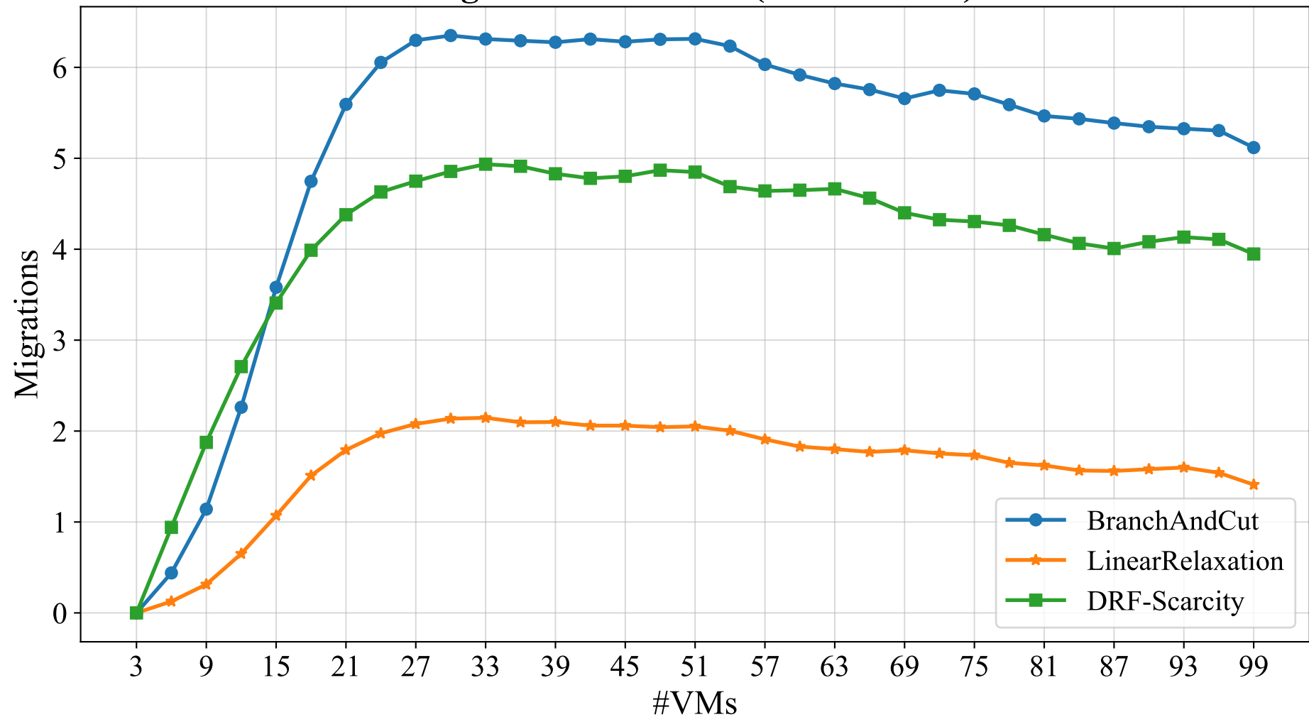
Migrations vs #VMs (over 3 Hosts)
