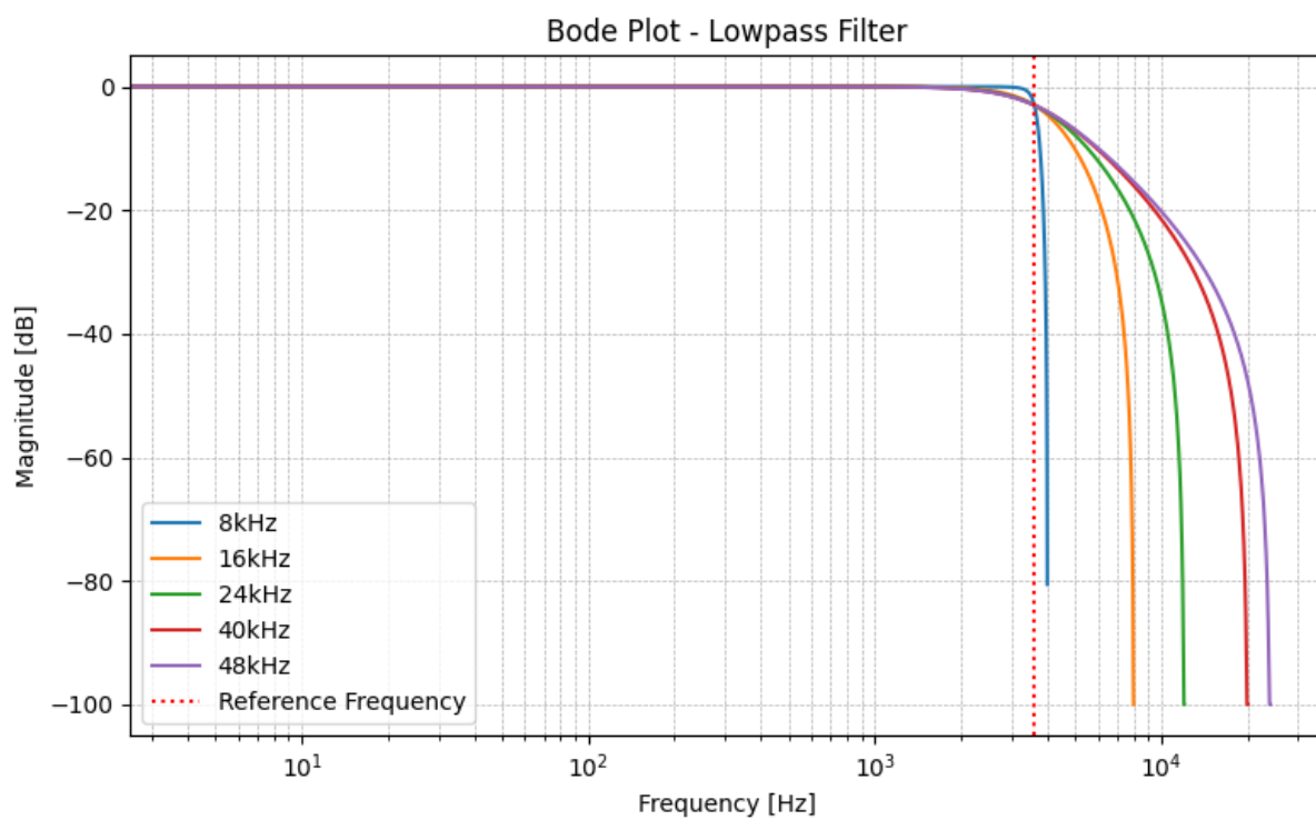
Figura 3: Diagrama de bode: Filtros pasa bajo
