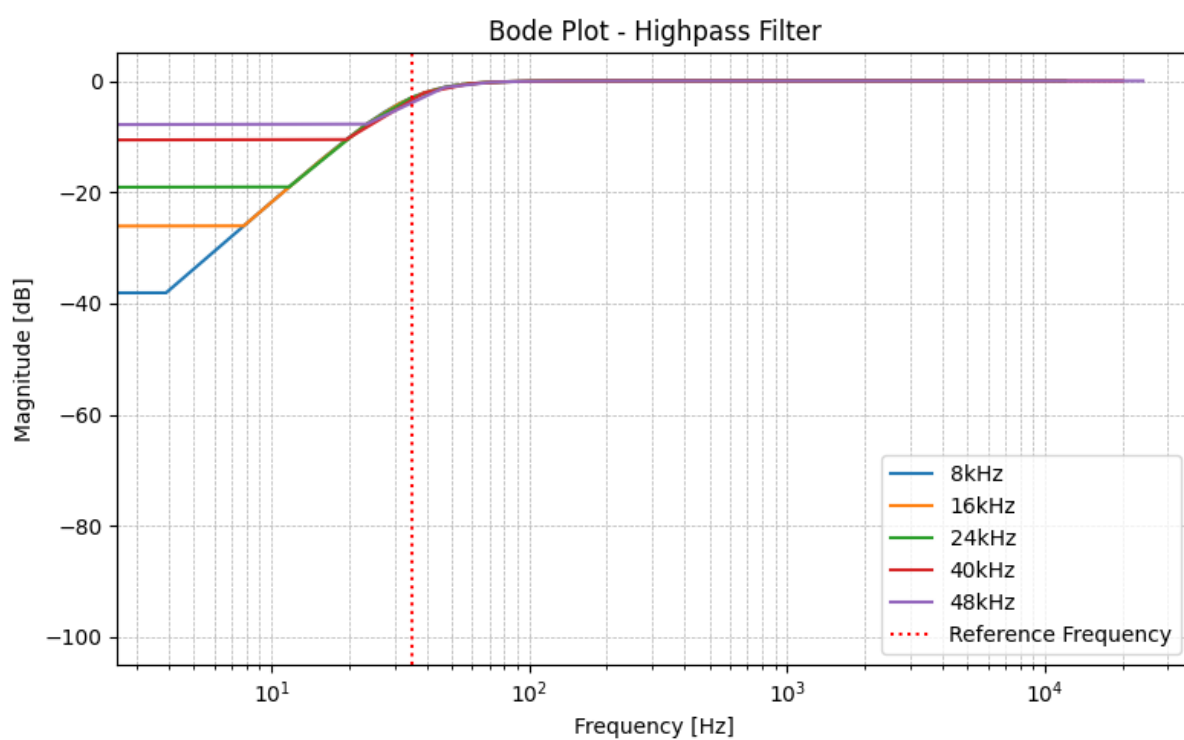
Figura 4: Diagrama de bode: Filtros pasa alto
