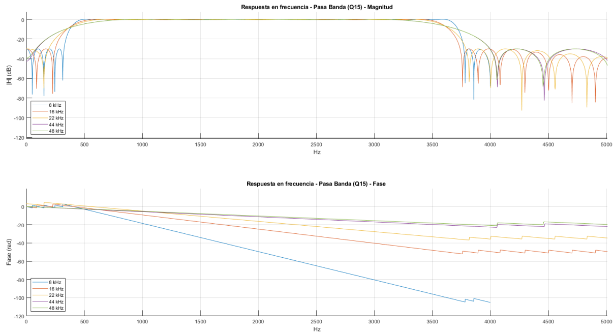
Figura 5: Respuesta en frecuencia de los filtros FIR pasa banda cuantizados en Q15
