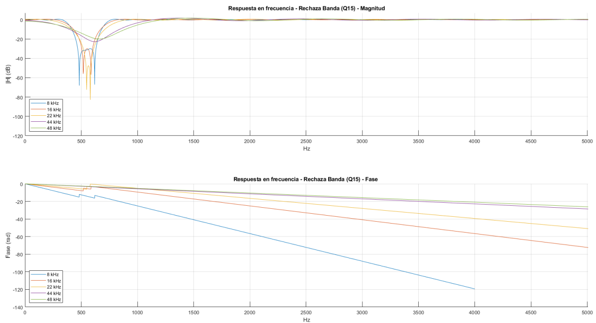
Figura 6: Respuesta en frecuencia de los filtros FIR rechaza banda cuantizados en Q15
