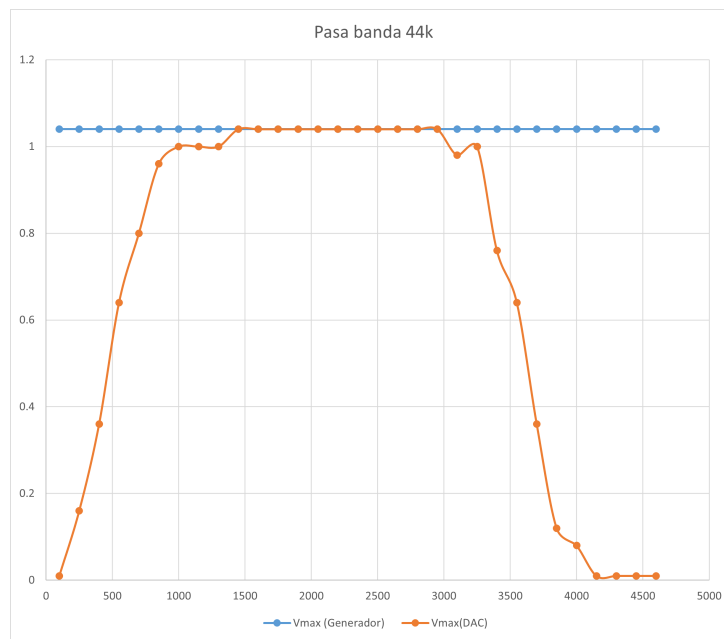
Figura 20: Respuesta en amplitud del filtro pasa banda para una frecuencia de muestreo de 44 kHz.
