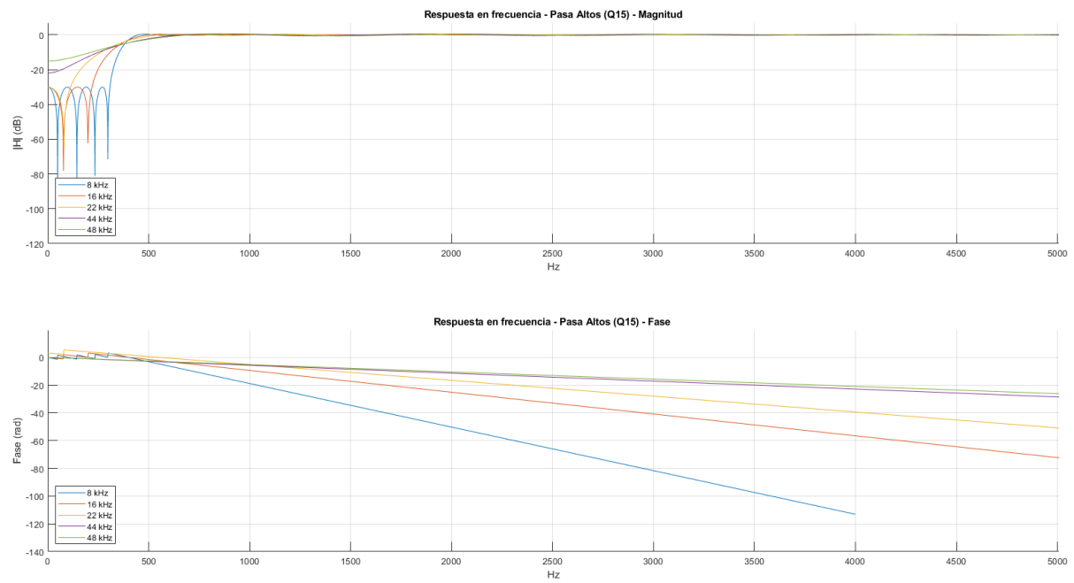
Figura 4: Respuesta en frecuencia de los filtros FIR pasa alto cuantizados en Q15
