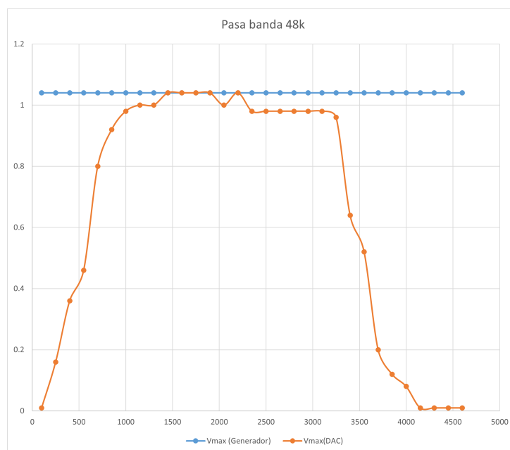
Figura 21: Respuesta en amplitud del filtro pasa banda para una frecuencia de muestreo de 48 kHz.
