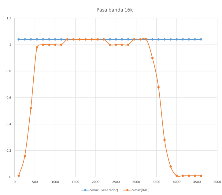
Figura 18: Respuesta en amplitud del filtro pasa banda para una frecuencia de muestreo de 16 kHz.
