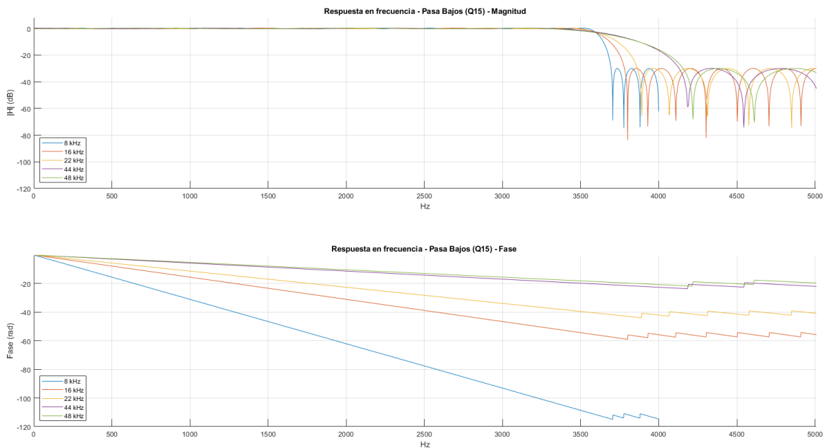
Figura 3: Respuesta en frecuencia de los filtros FIR pasa bajo cuantizados en Q15
