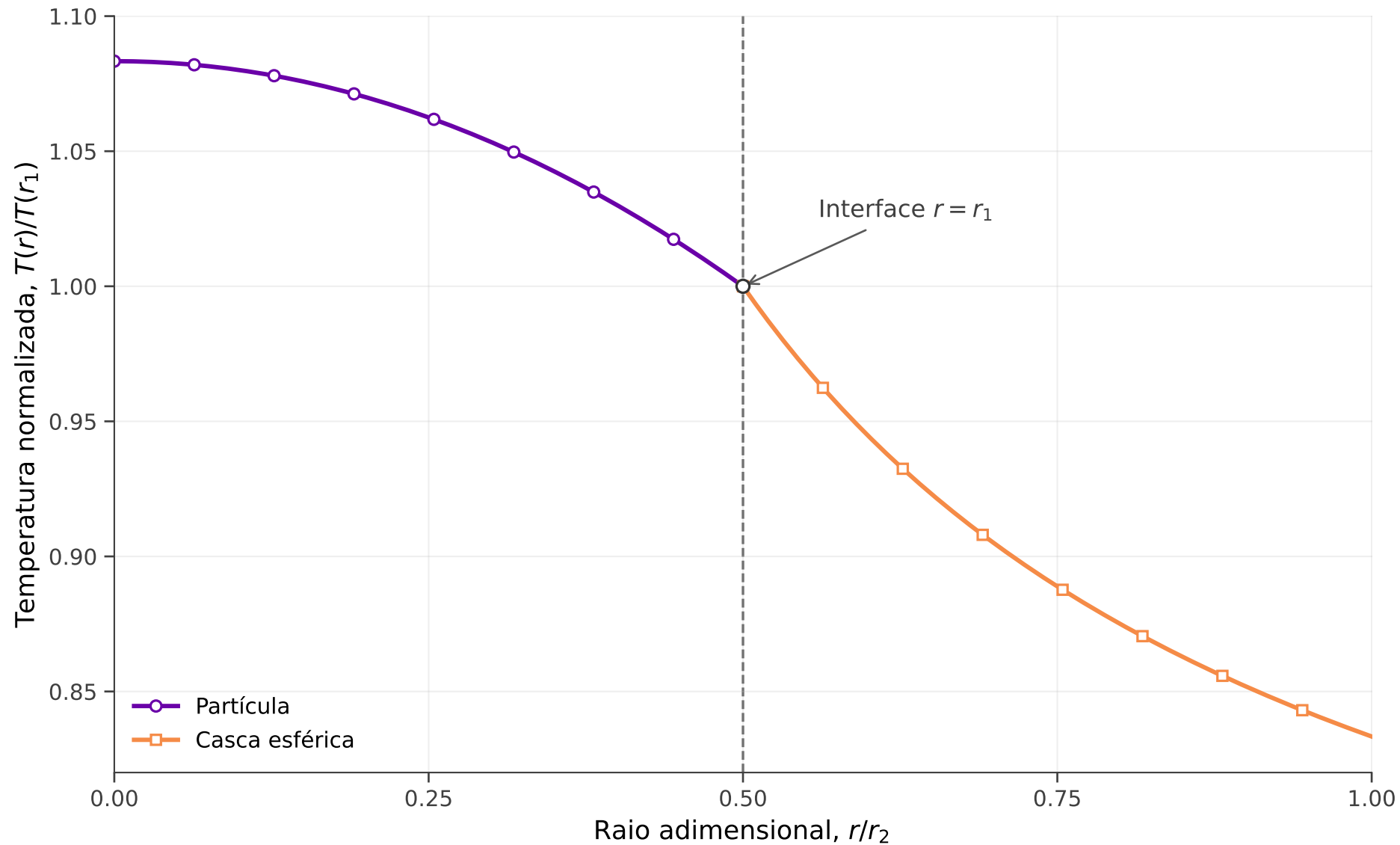
Distribuição de temperatura: r_1/r_2 = 0,5 e k_1 = 2k_2
