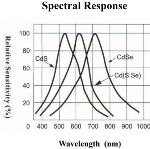
Figura 2: Respuesta espectral del LDR GL5528 según su hoja de datos.
