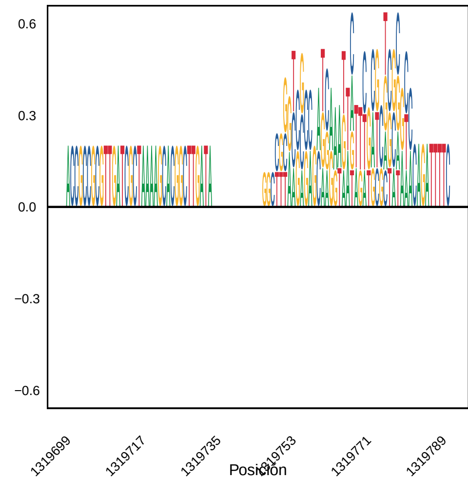
ROI 3 (1319699 – 1319790)
