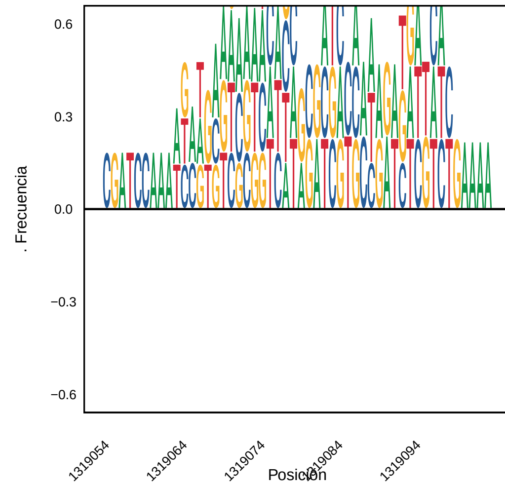
ROI 1 (1319054 – 1319103)
