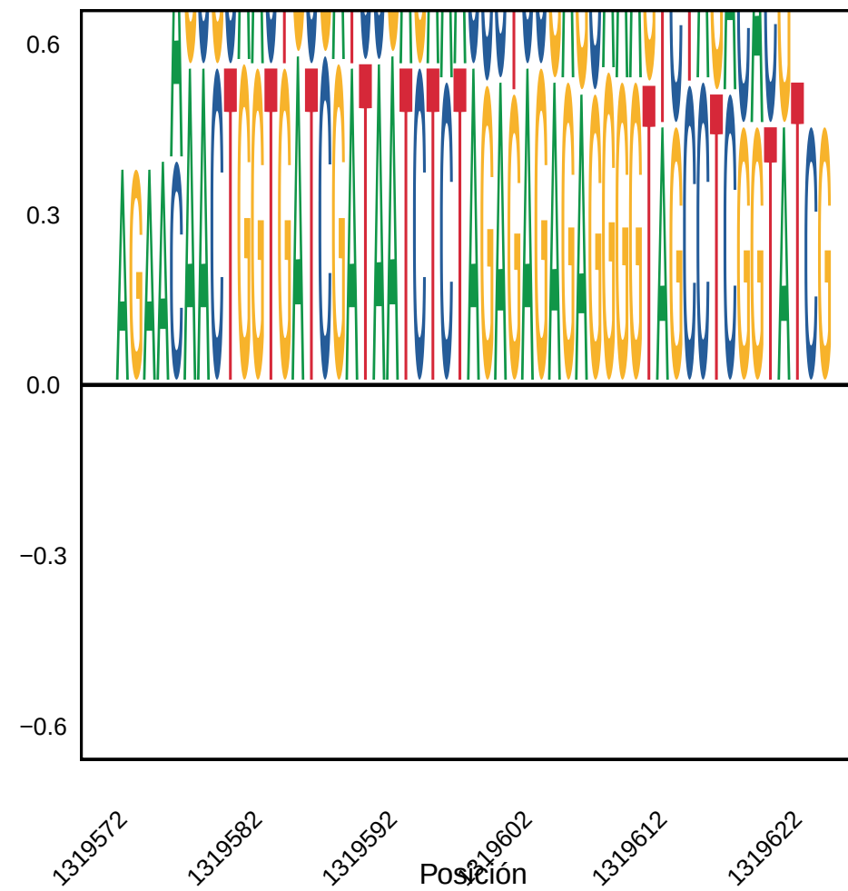
ROI 2 (1319572 – 1319624)
