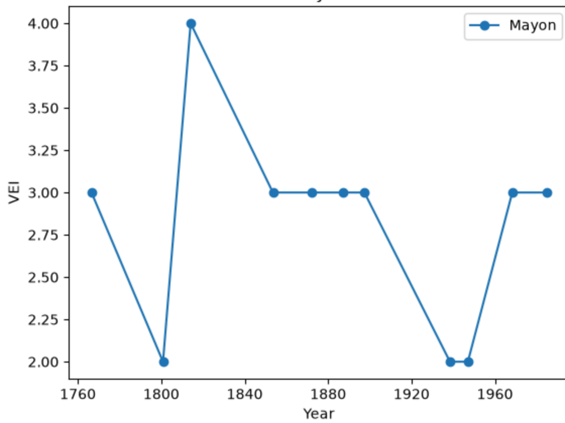
Mayon
