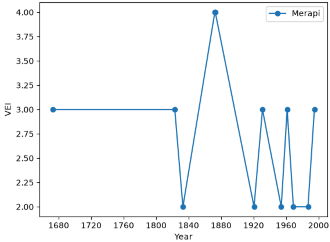
Merapi
