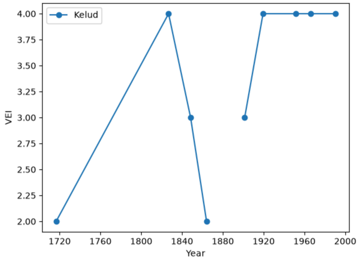
Kelud
