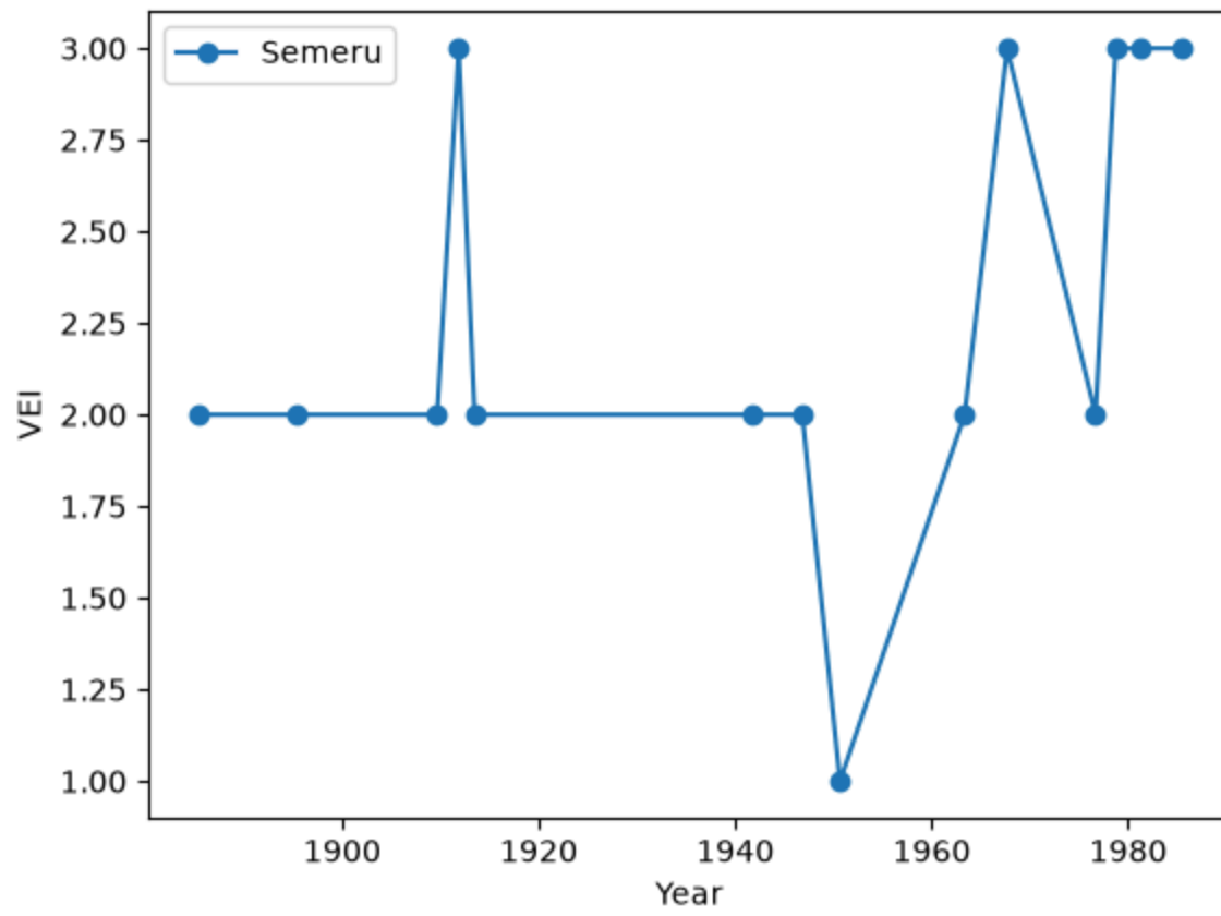
Semeru
