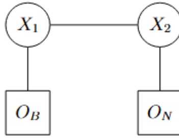
Figura 4.1: Modelo Oculto de Markov para un píxel con dos estados ocultos y dos observaciones.
