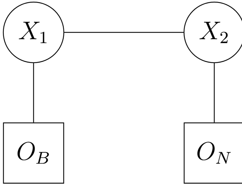
Figura 7.1: Modelo Oculto de Markov para un píxel con dos estados ocultos y dos observaciones.
