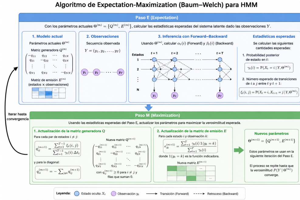
Figura 8.1: Esquema general del algoritmo Expectation–Maximization (Baum–Welch) para un Modelo Oculto de Markov. En el Paso E se estiman las probabilidades posteriores de los estados ocultos y las transiciones esperadas mediante los algoritmos Forward–Backward. En el Paso M se actualizan iterativamente la matriz generadora y la matriz de emisión para maximizar la verosimilitud de las observaciones.
