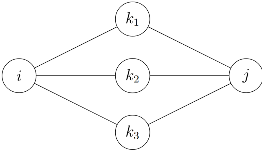
Figura 4.1: La probabilidad de transición p_{ij}(t + s) se obtiene sumando las contribuciones de todos los posibles estados intermedios k .
