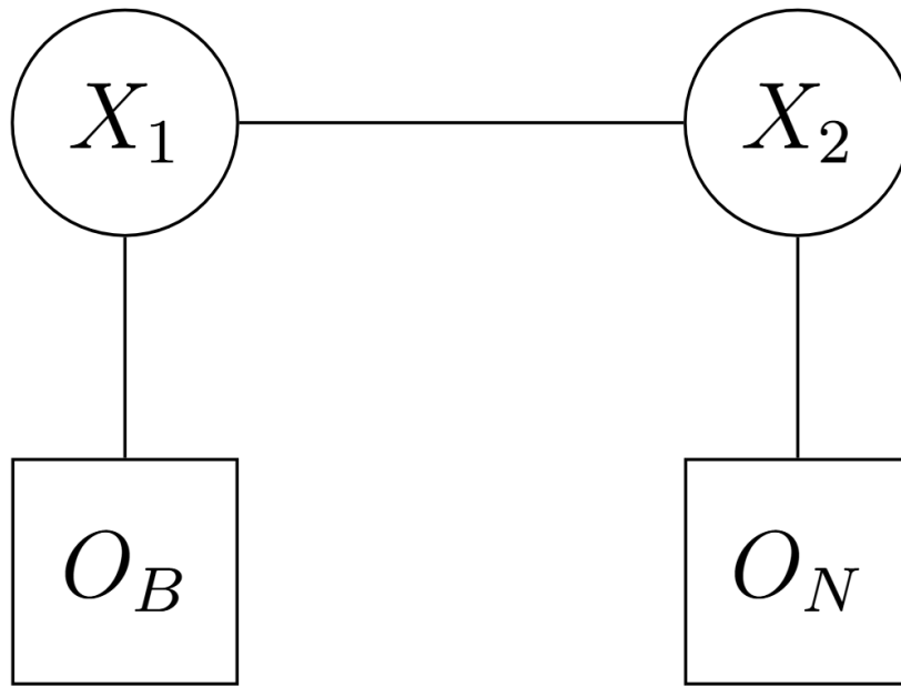
Figura 16.1: Modelo Oculto de Markov para un píxel con dos estados ocultos y dos observaciones.
