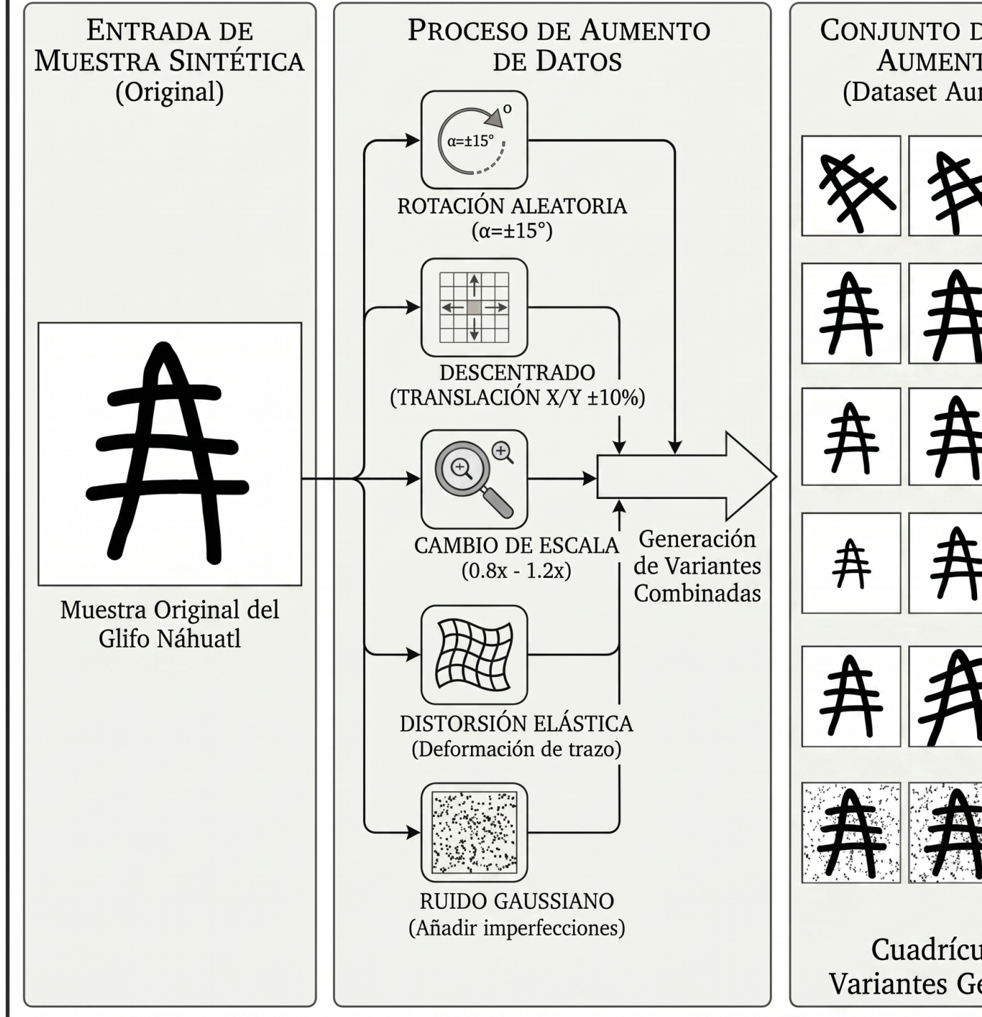
Figura 19.2: Se observa el proceso por el que pasa cada una de las 25 imágenes por letra para generar 90 variantes obtenidas a partir de rotación, traslación, distorsión elástica, cambio de escala y ruido, de este modo se consigue un dataset más completo.
