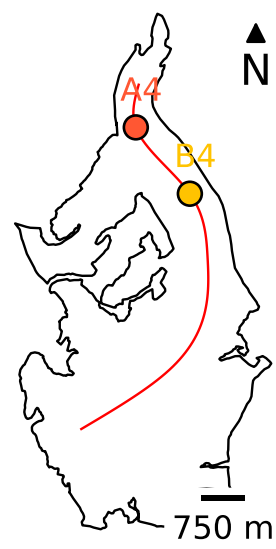
Corbassière
