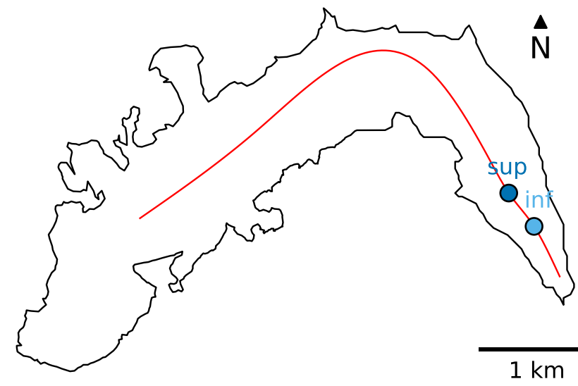
Glacier Blanc
