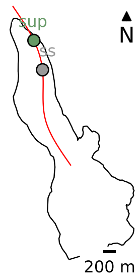
Gébroulaz
