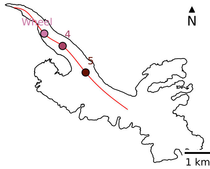
Argentière
