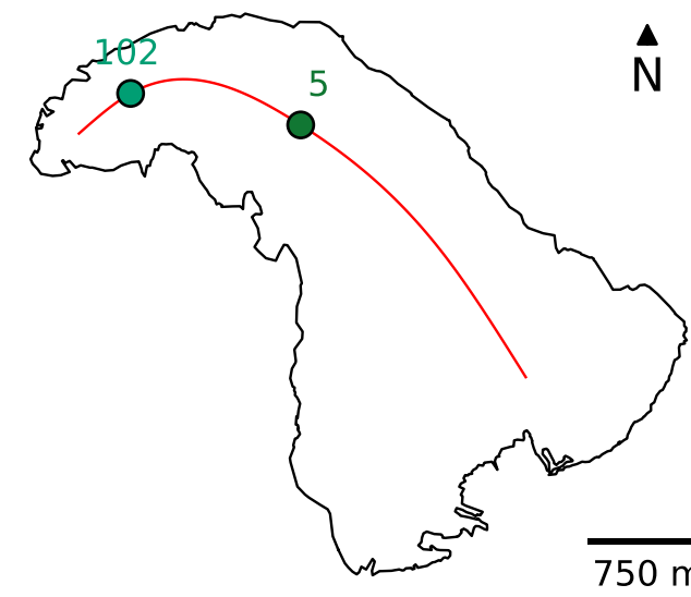
Giétro
