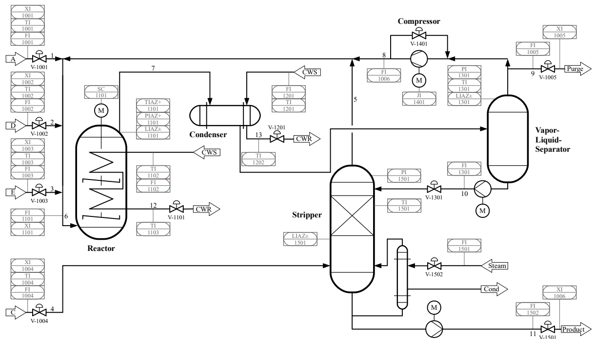
Abbildung 3.12: Anlagenschema des TEP mit seinen fünf Hauptkomponenten, in Anlehnung an [BRJ15], in Schwarz vereinheitlicht
