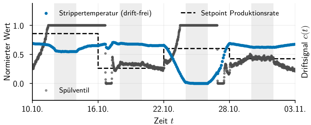
(a) Betriebspunkte
