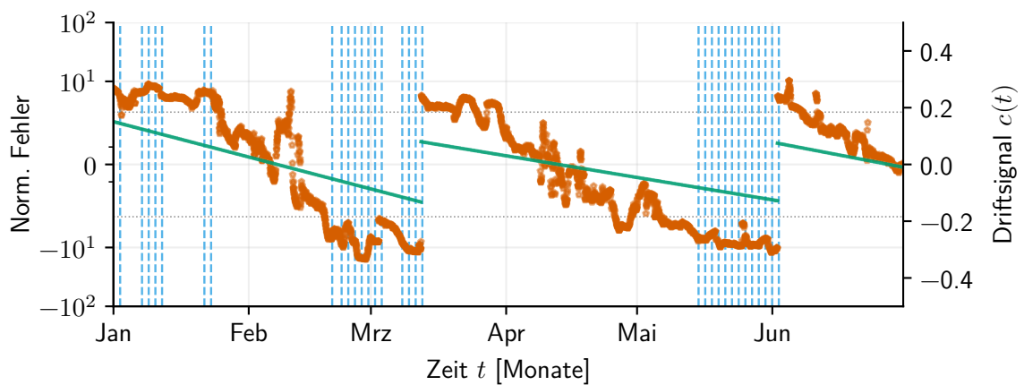
(c) Schwellwert-Detektor
