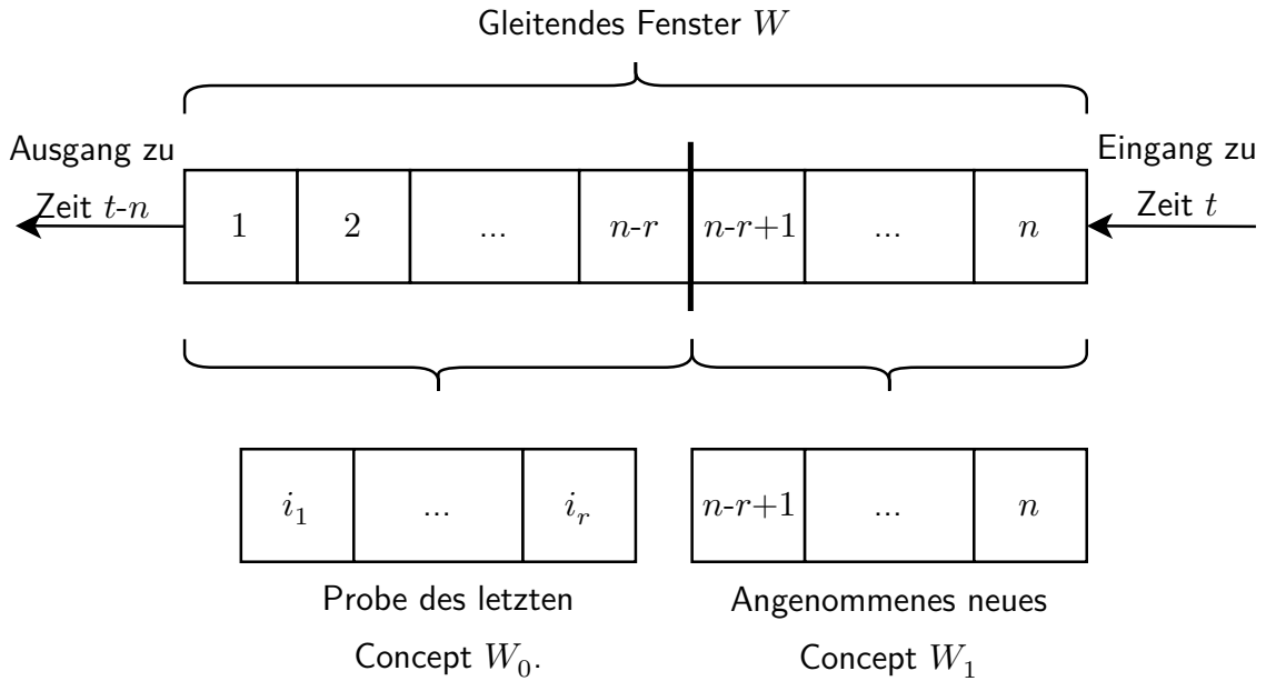
Abbildung 2.7: Speicherstrategie von Kolmogorov-Smirnov Windowing (KSWIN) angelehnt an [RHS20]
