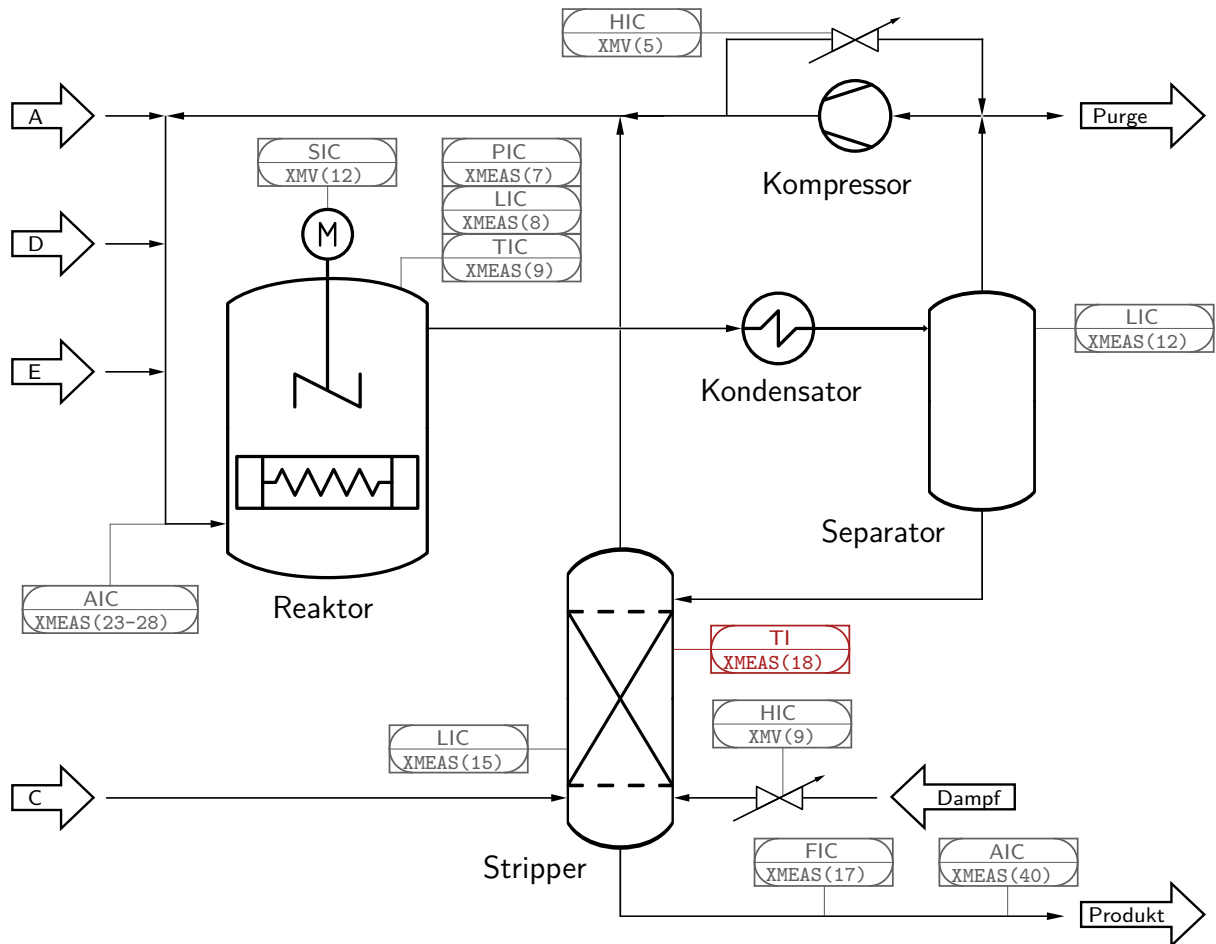
Abbildung 3.12: Anlagenschema des TEP mit seinen fünf Hauptkomponenten, nach [DV93]; in Grau: Setpoints aus Tabelle A.2, in Rot: Strippertemperatur XMEAS(18)
