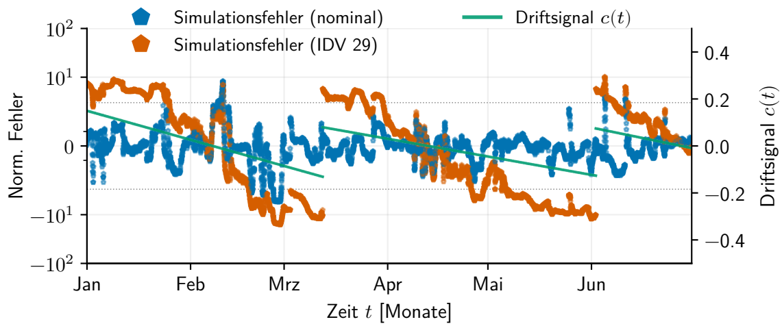
Abbildung 3.14: Normierter Simulationsfehler auf dem nominalen und dem drift-behafteten Datenstrom im Vergleich zum Driftsignal c(t)
