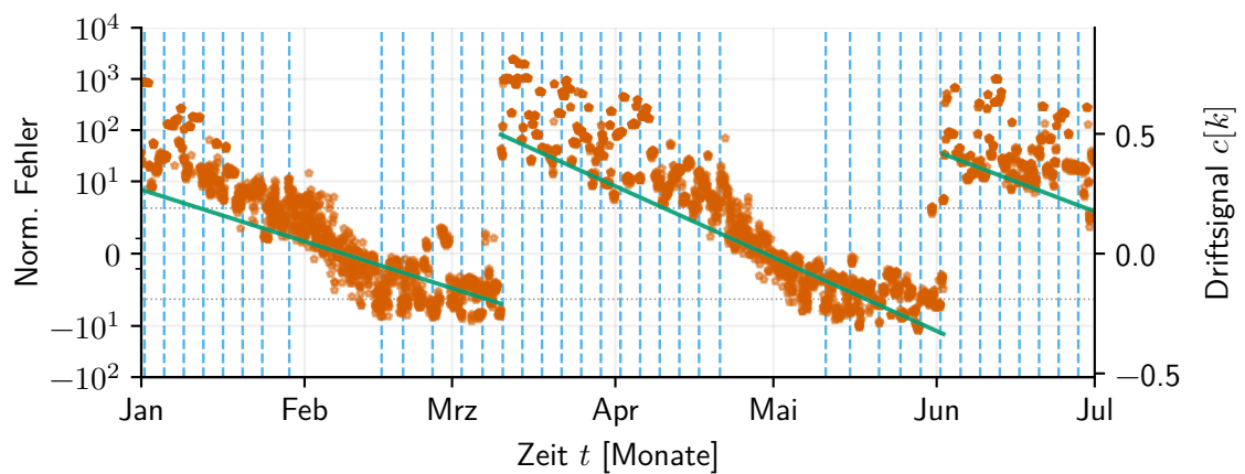
(c) Schwellwert-Detektor
