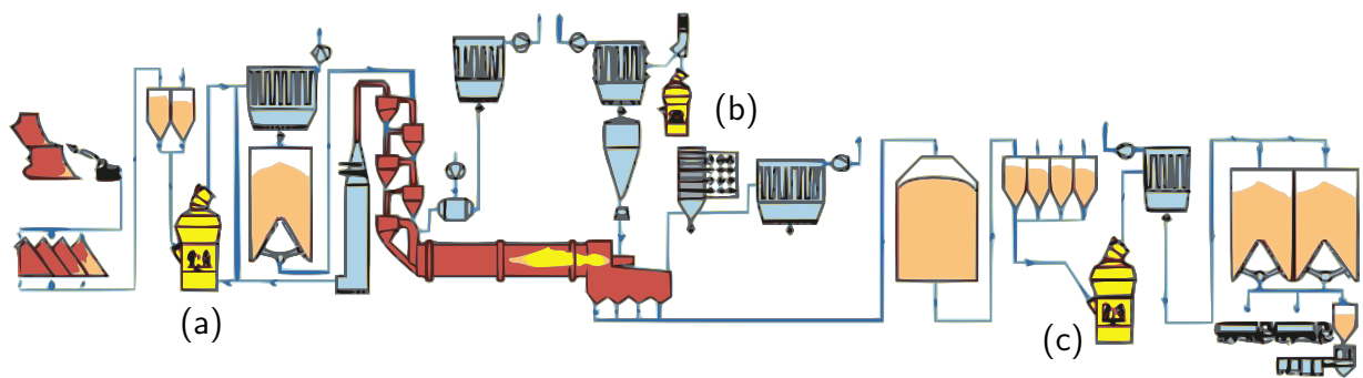
Abbildung 2.1: Schematische Abbildung der konsektiven Prozessschritte in der Zementherstellung, Abbildung von Gebr. Pfeiffer SE
