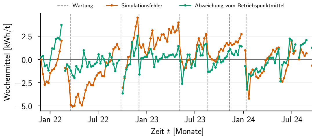
Abbildung 4.3: Wochenmittel von Driftsignal und Simulationsfehler
