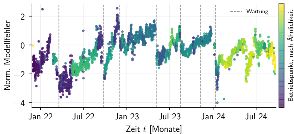
Abbildung 4.5: Normierter Simulationsfehler nach Betriebspunkt
