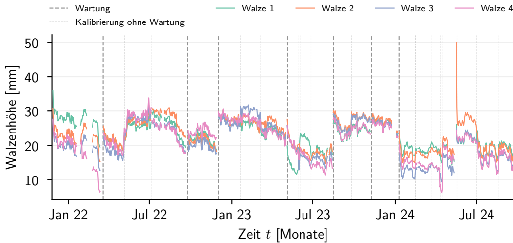
Abbildung 4.4: Gemessene Höhe der vier Walzen mit den Wartungen
