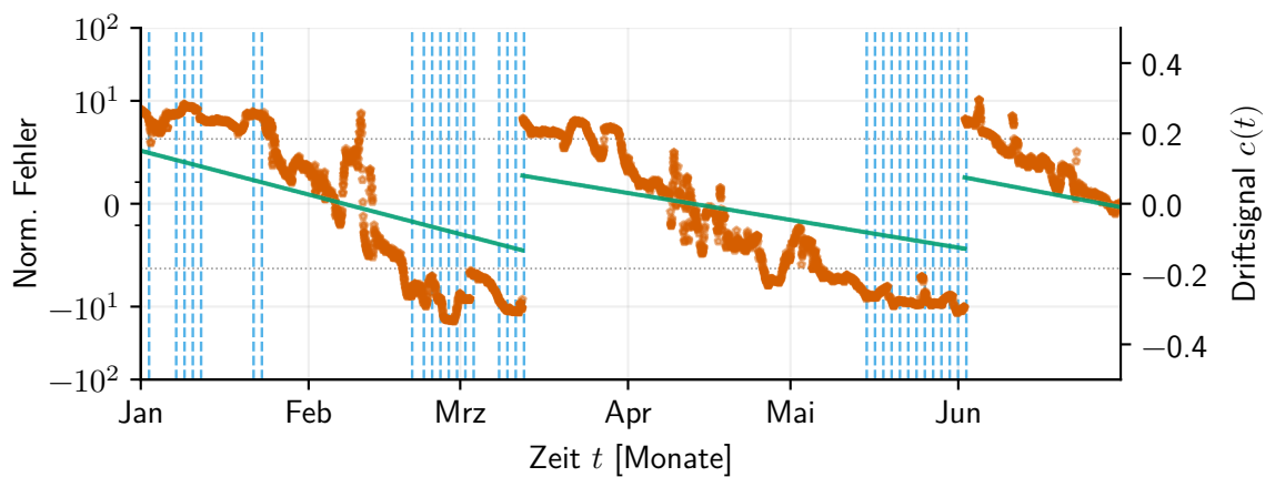
(c) Schwellwert-Detektor
