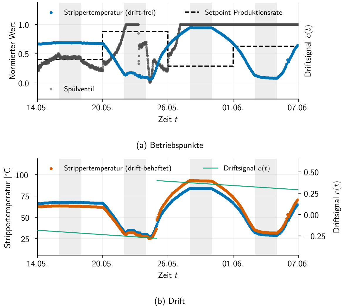
Abbildung 3.13: Ausschnitt des erzeugten Datenstroms über vier Betriebspunkte.
