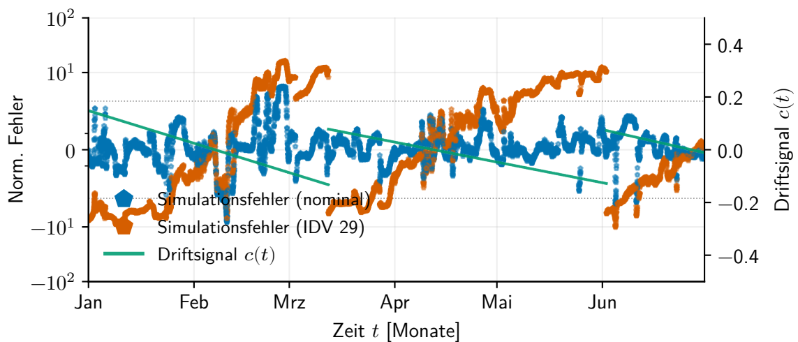
Abbildung 3.14: Normierter Simulationsfehler auf dem nominalen und dem drift-behafteten Datenstrom im Vergleich zum Driftsignal c(t)
