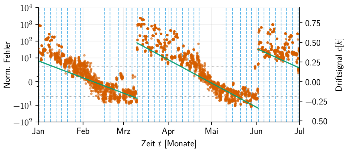
(c) Schwellwert-Detektor
