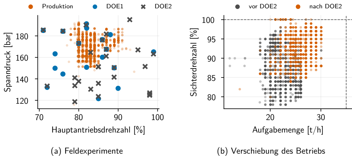
Abbildung 4.2: Abdeckung des Stellgrößenraums
