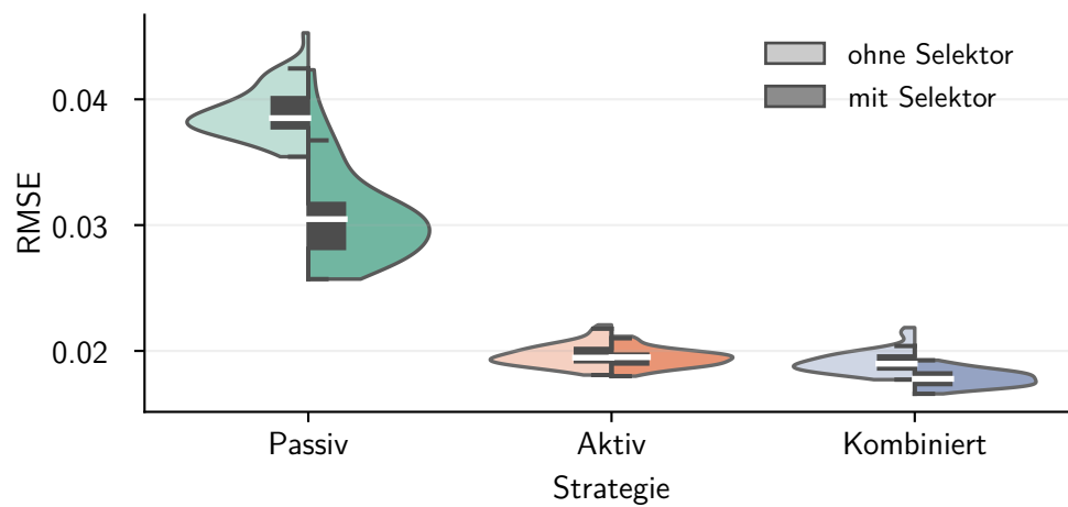
Abbildung 3.18: Verteilung des RMSE der adaptiven Strategien über 50 Läufe mit unterschiedlichen Seeds
