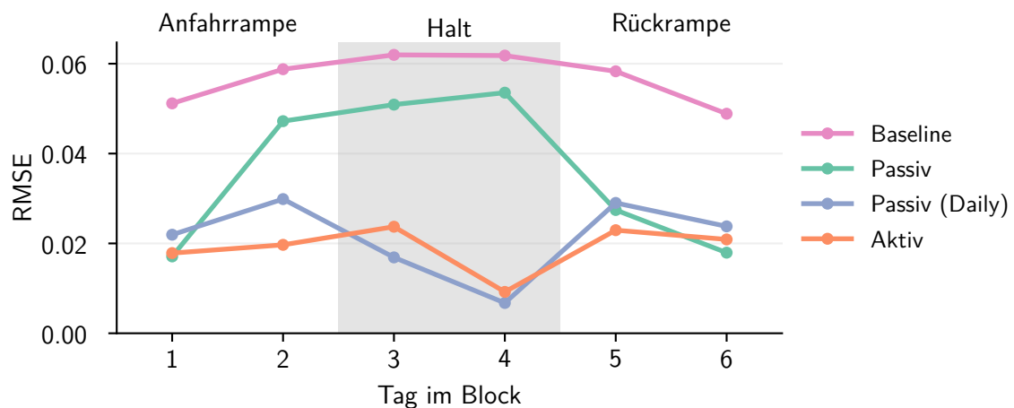
Abbildung 3.16: Mittlerer RMSE je Tag eines Betriebspunkt-Blocks über 50 Seeds
