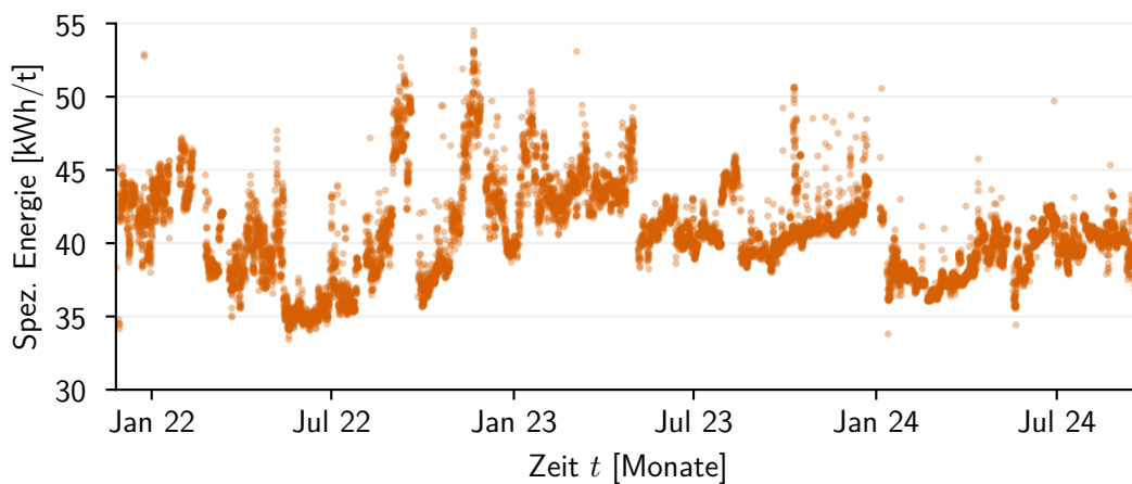
Abbildung 4.1: Spezifische Energie der Betriebspunkte im Produktionsbetrieb
