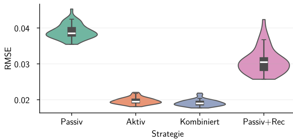
Abbildung 3.17: Verteilung des RMSE der adaptiven Strategien über 50 Läufe mit unterschiedlichen Seeds
