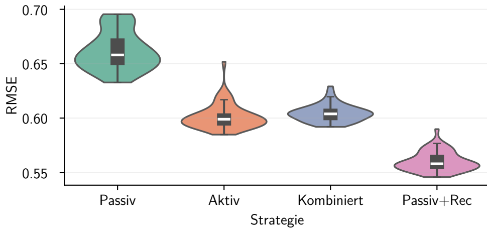
Abbildung 3.11: Verteilung des RMSE der vier adaptiven Strategien über 50 Läufe mit unterschiedlichen Seeds, dargestellt als Violinen mit überlagerten Boxplots
