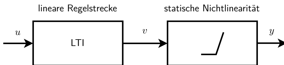
Abbildung 3.6: Struktur des Wiener-Modells
