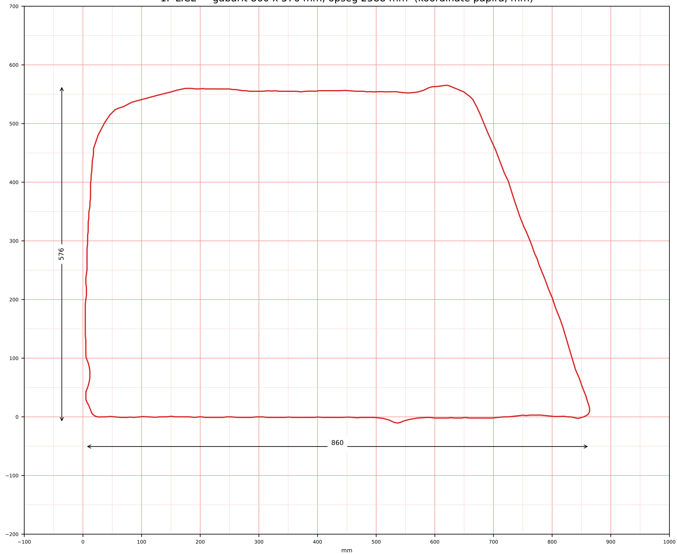
1F LICE - gabarit 860 x 576 mm, opseg 2588 mm (koordinate papira, mm)
