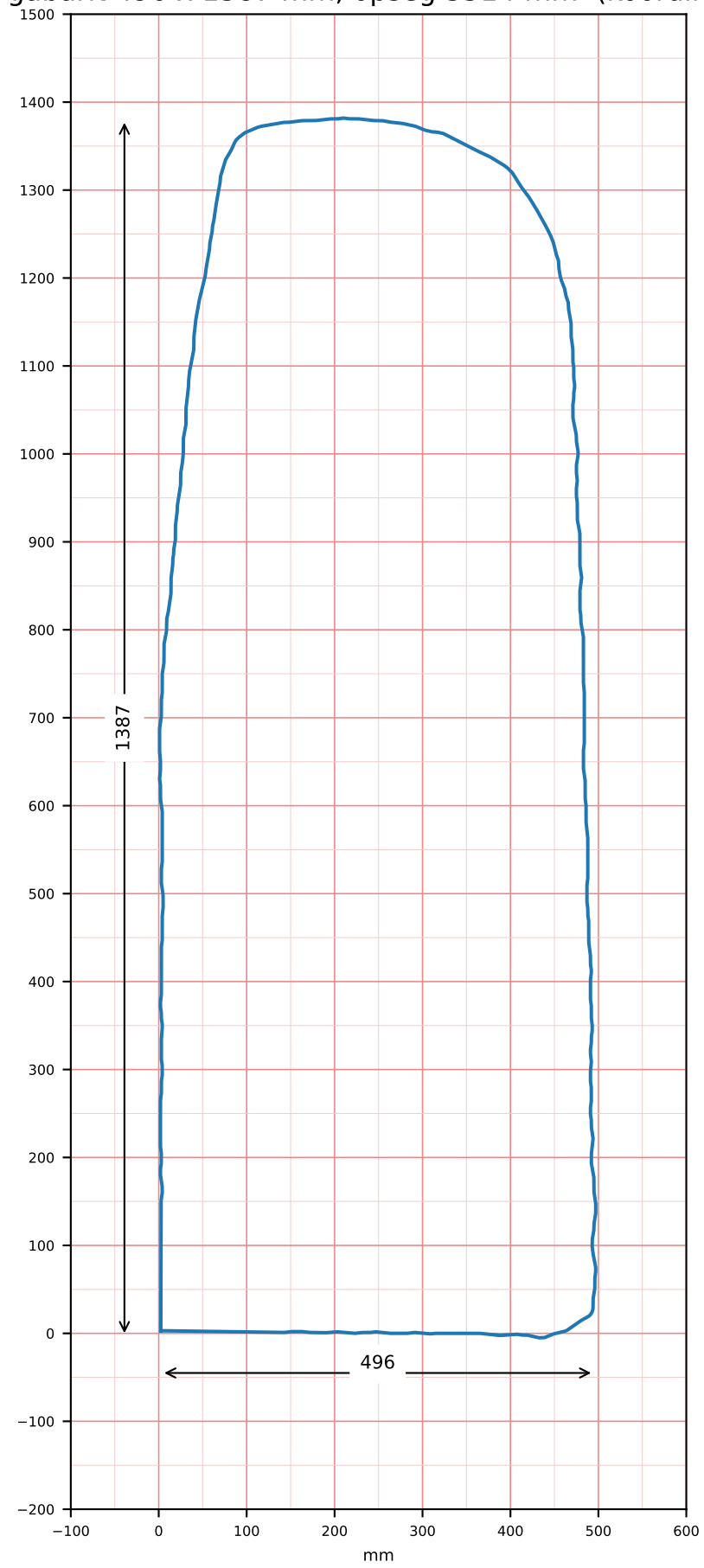
KLUP LICE - gabarit 496 x 1387 mm, opseg 3514 mm (koordinate papira, mm)
