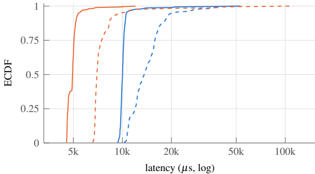
GEMM 512
