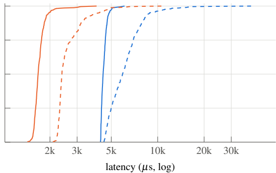
Kalman 32768
