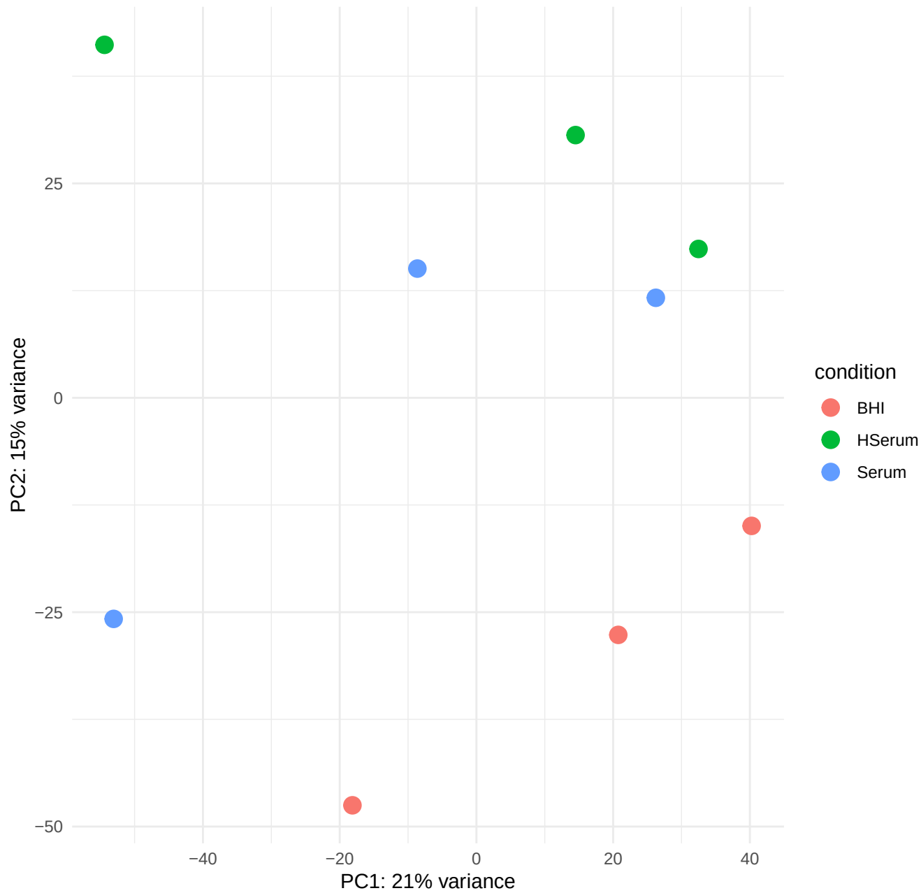
PCA of TnSeq samples (Serum, HSerum, BHI)
