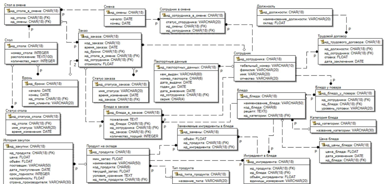
Рисунок 1 – Схема инфологической модели данных БД в нотации IDEF1X
