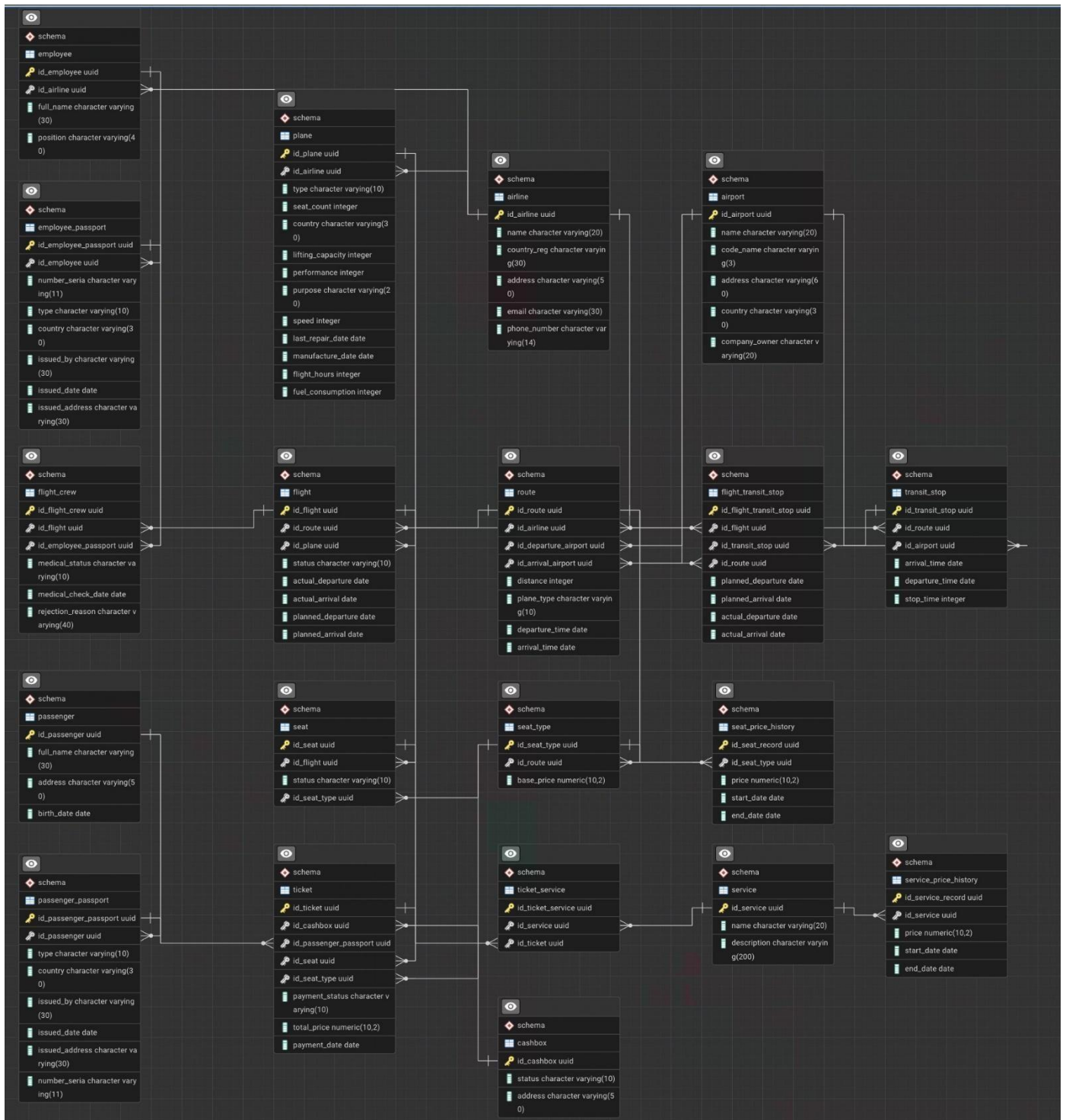
Рис. 2: ERD-диаграмма БД «Аэропорт»
