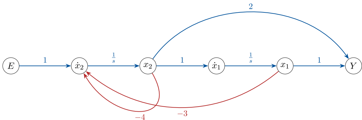
图 4: 题 22: 二阶系统信号流图
