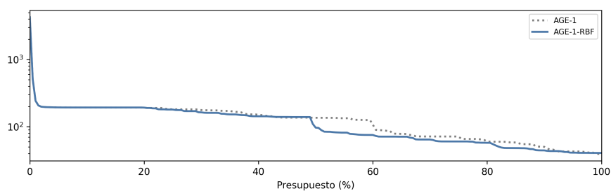
(b) f_9
