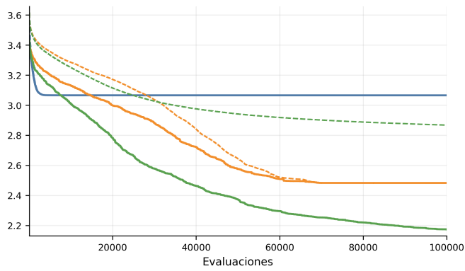
(b) f_{10}
