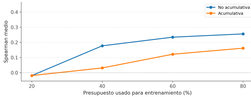
(b) DE
