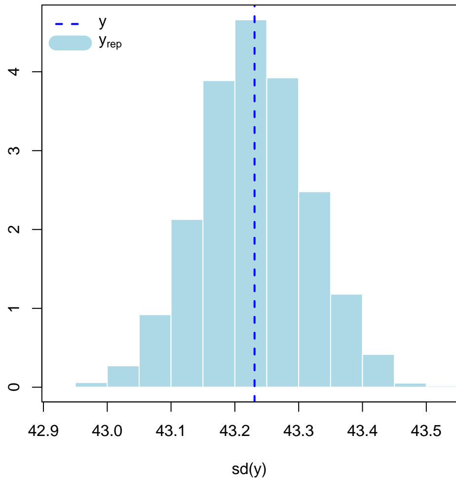
Posterior predictive std. dev.
