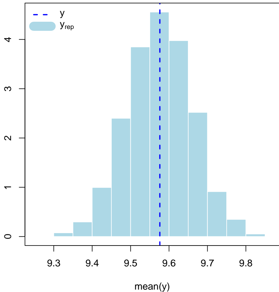
Posterior predictive mean
