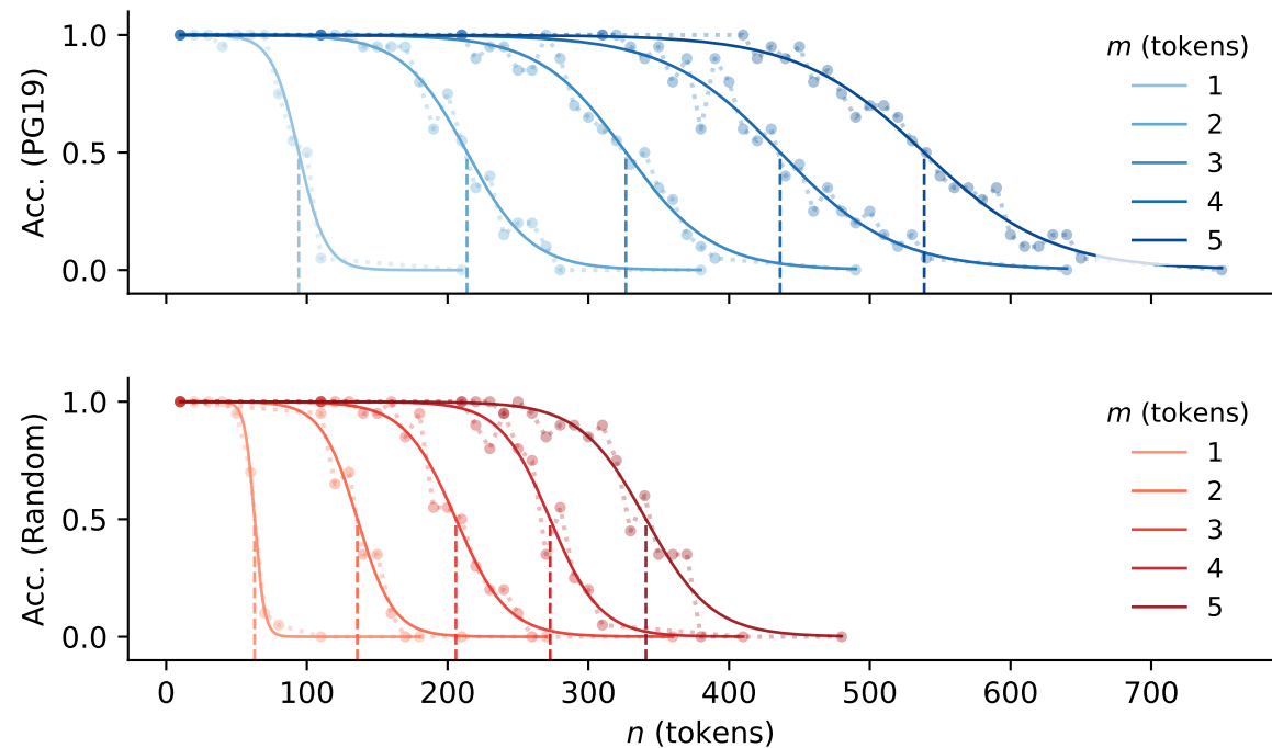
Pythia-410m
