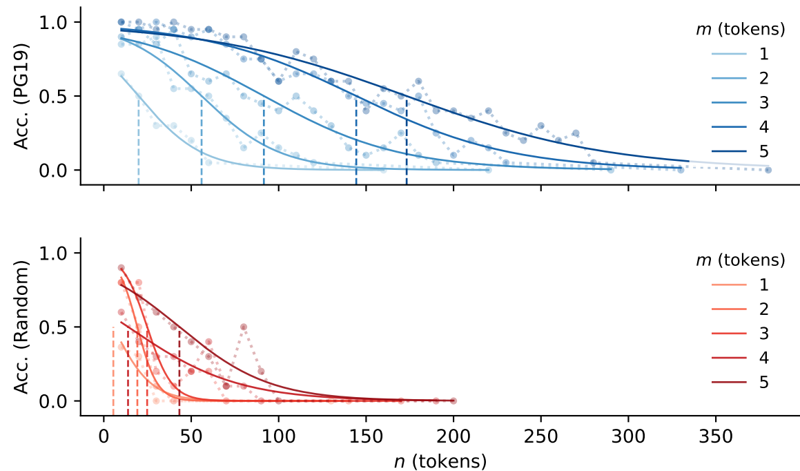
Gemma-3-1b-pt
