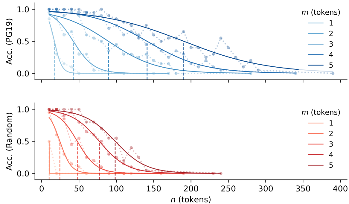
Gemma-3-270m
