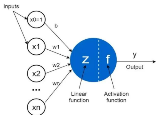
Percettrone, 1957
