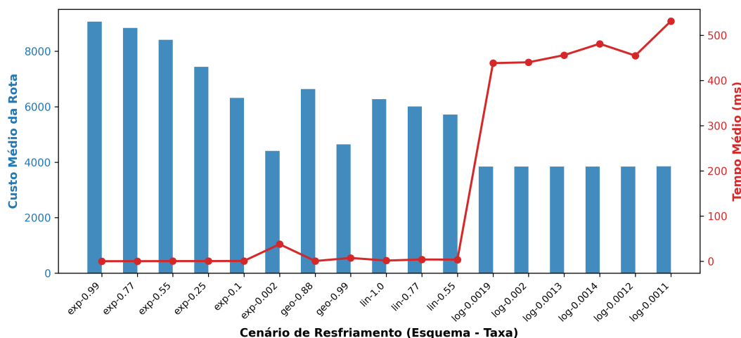
Figura 1: Relação entre Taxa de Resfriamento, Custo Final e Tempo Médio na TS
