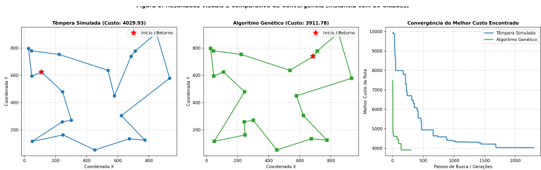
Figura 1. Resultados na instância de 20 cidades: rota final da Têmpera Simulada (esquerda), rota final do Algoritmo Genético (centro) e curvas de convergência de custo por iteração (direita).
