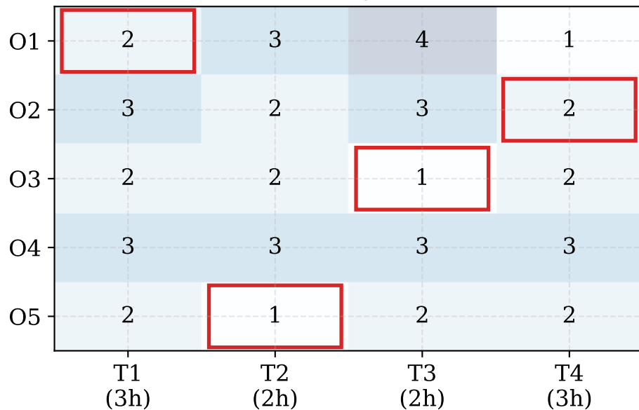
Solución Óptima | Coste Total: 6
