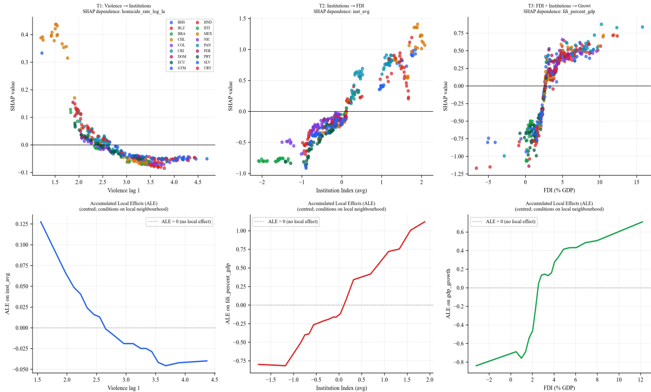
Efectos marginales acumulados (ALE) y valores SHAP para los predictores clave.
