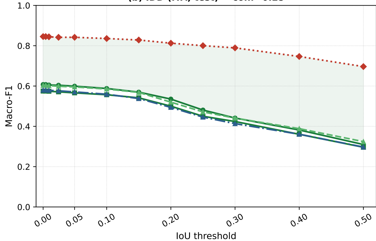
(b) IDD (ITA, test) -- conf=0.25
