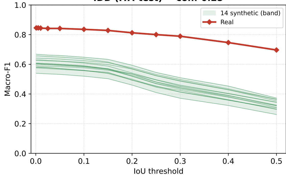
IDD (ITA-test) -- conf 0.25
