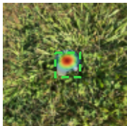
YOLOv11l real
