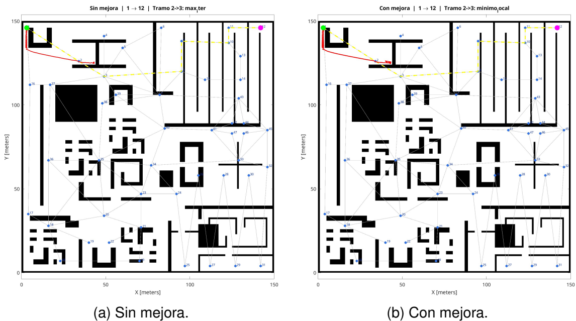
Figura 1: Caso base nodo 1 \rightarrow nodo 12 con planificación global Dijkstra y navegación local por campos potenciales sobre mapa2.pgm . Aristas del grafo en gris, ruta global en amarillo discontinuo, trayectoria del robot en rojo, origen verde y destino magenta.
