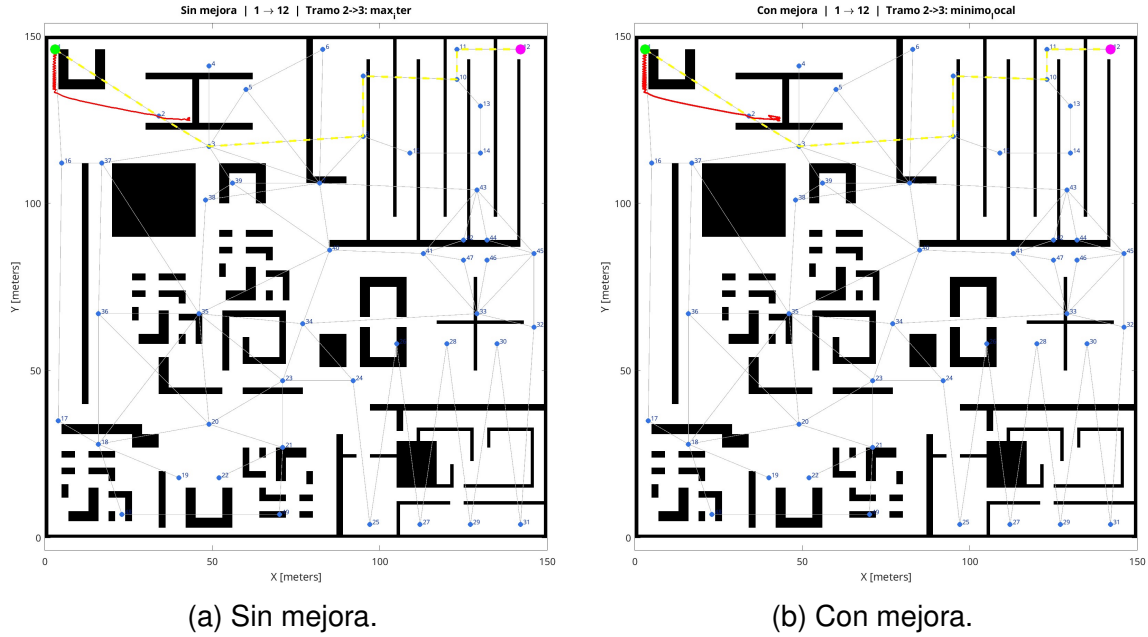
Figura 7.1: Caso base nodo 1 \rightarrow nodo 12 con planificación global Dijkstra y navegación local por campos potenciales sobre mapa2.pgm . Aristas del grafo en gris, ruta global en amarillo discontinuo, trayectoria del robot en rojo, origen verde y destino magenta.
