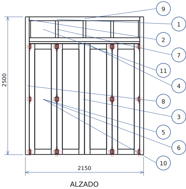
ALZADO
