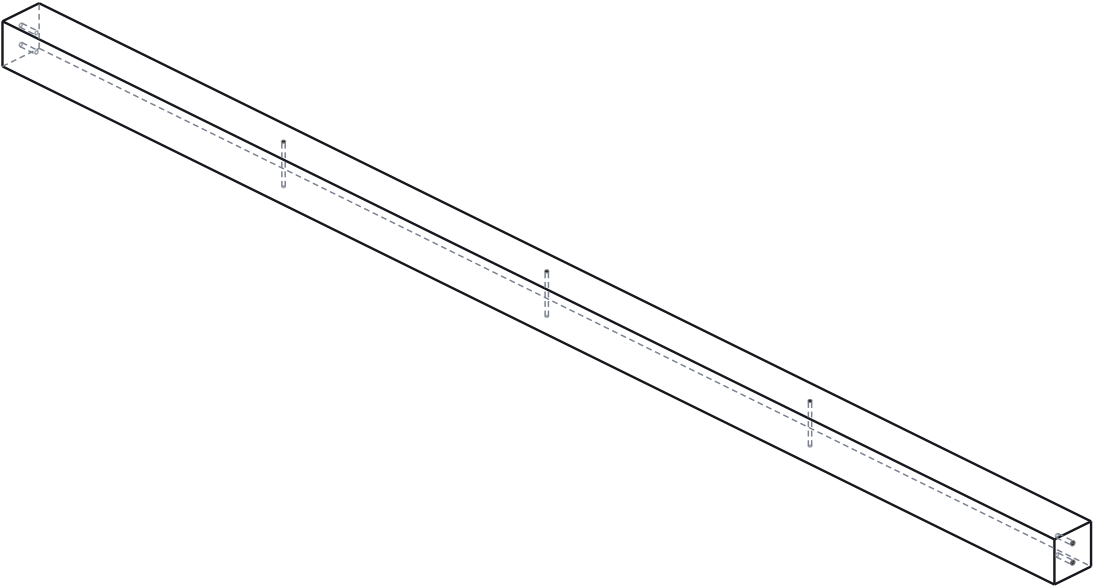
ISOMÉTRICA (sin escala)
