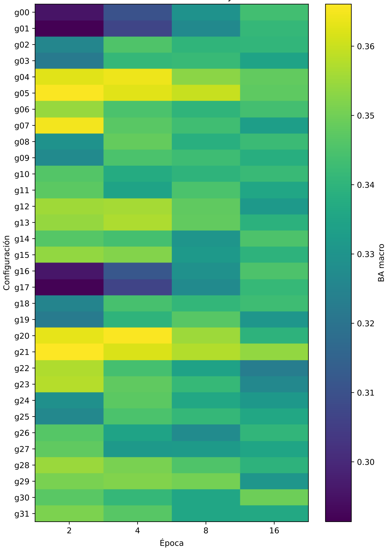
LSTM: BA interna media sobre folds y suavizados
