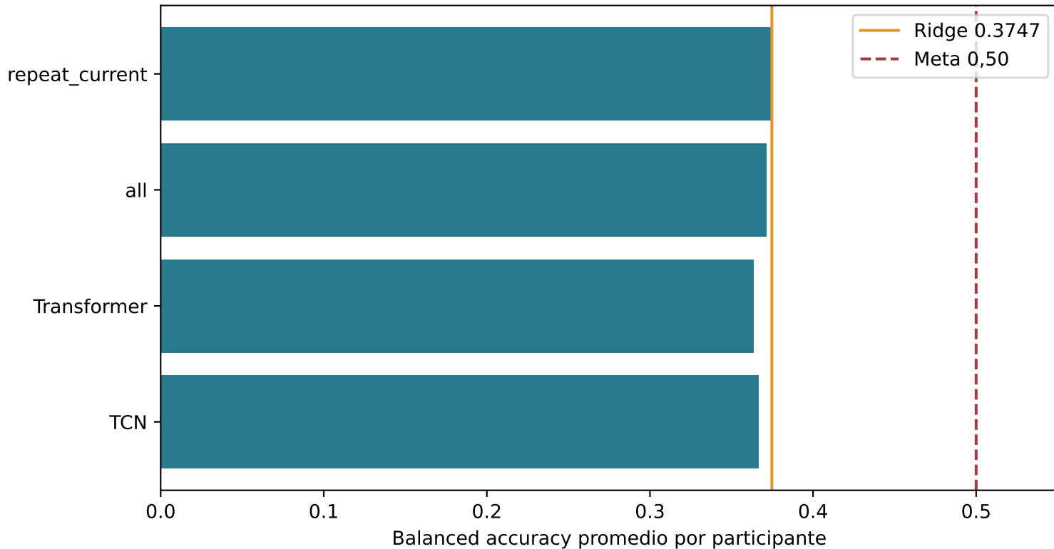
Transformer y TCN: evaluación exploratoria en train
