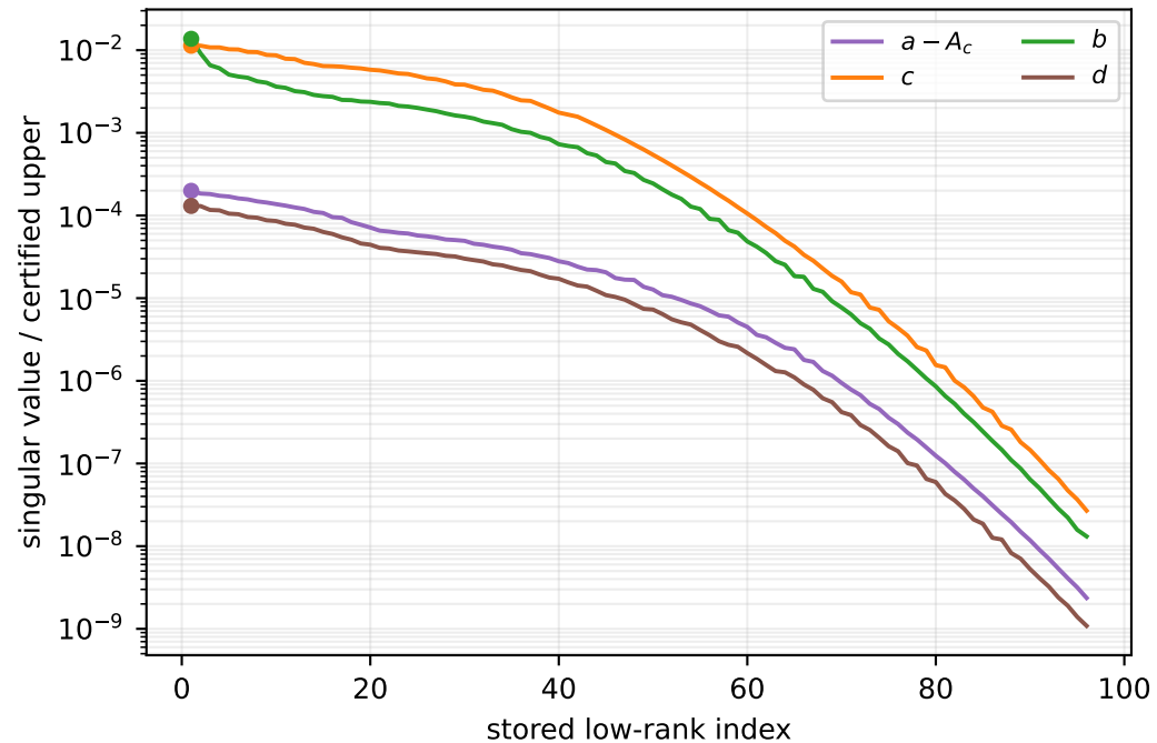
(d) Nested-grid continuation product
