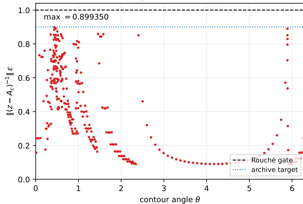
(d) Nested-grid continuation product
