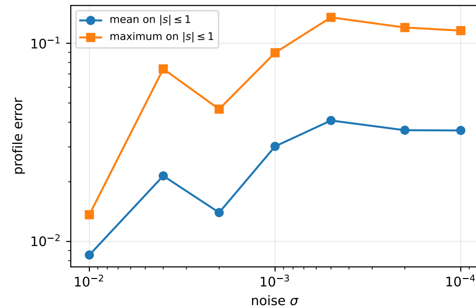
(d) Recentered archived cloud audit
