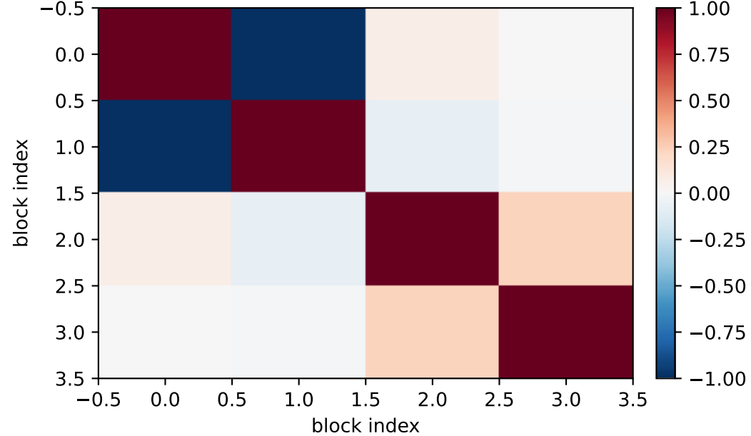
(d) Right normalized block Gram at \sigma = 0.01
