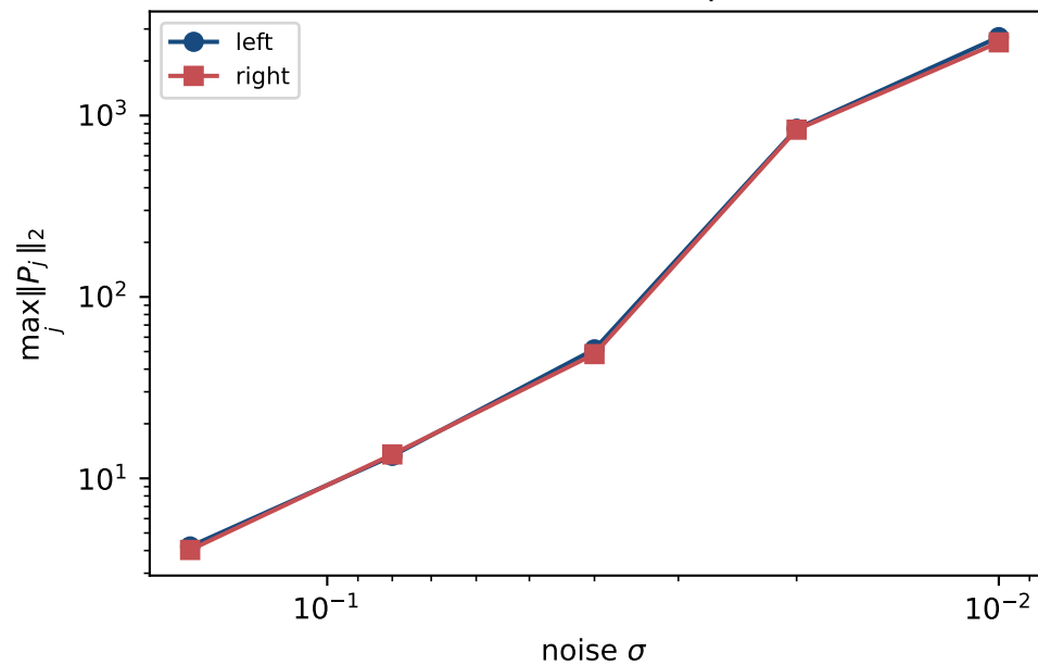
(b) Radial Riesz obliqueness
