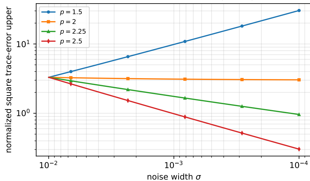
(d) Anchored bulk retains the p > 2 gate
